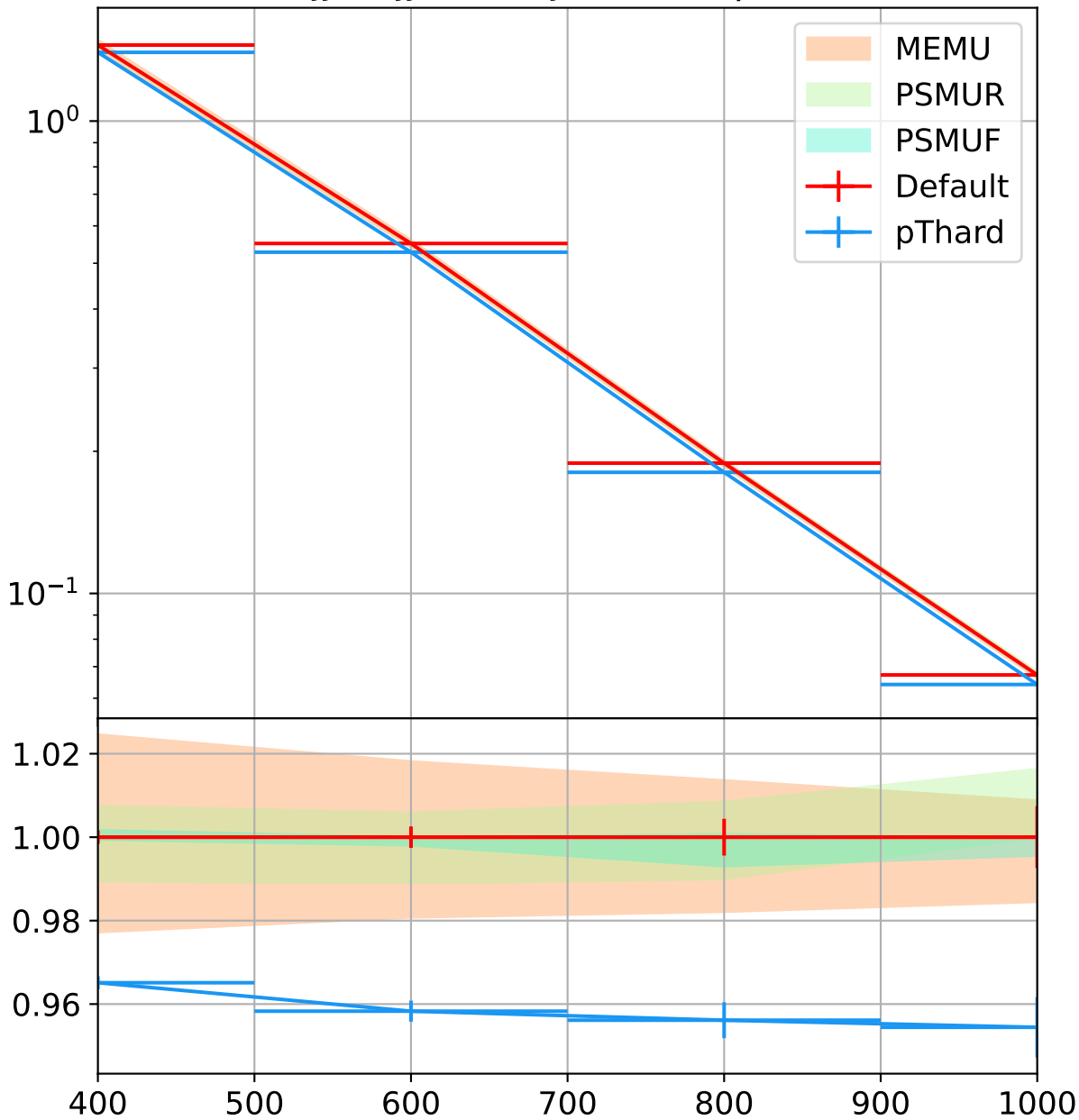
HISTO-MJJ-DYJJ-2-4-PTJ-30, Sherpa default PS
