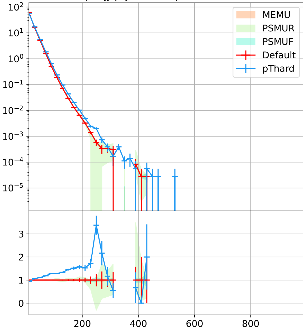
ptHjj-ptj30, Sherpa default PS
