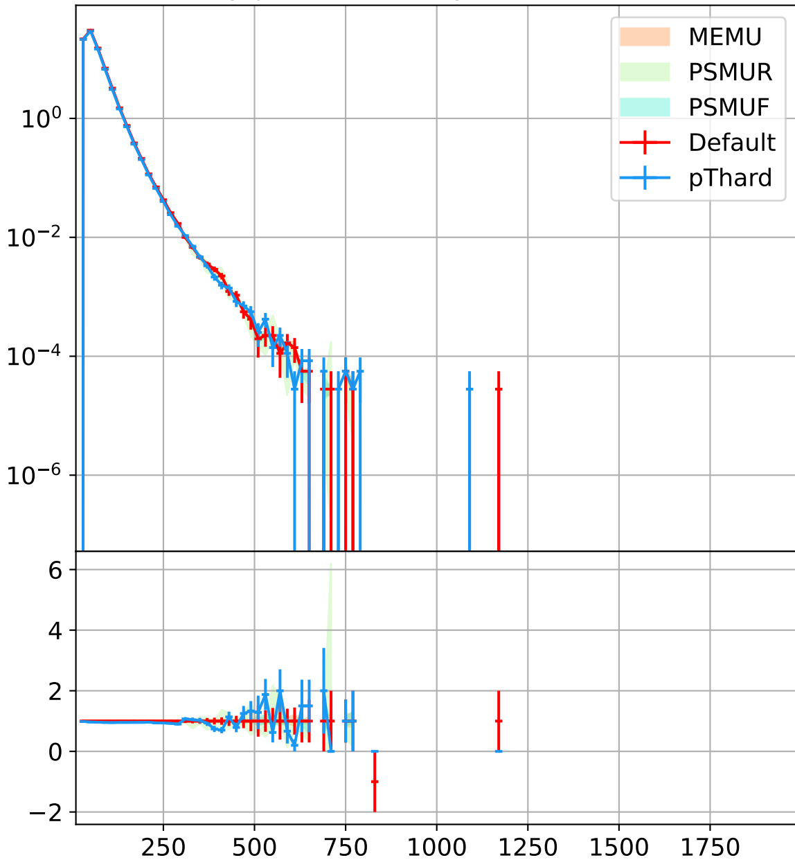
ptj2-STXS, Sherpa default PS
