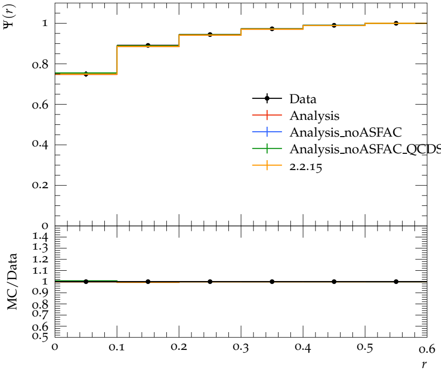
Jet shape \Psi for p_{\perp} \in 310\text{--}400\text{ GeV} , y \in 0.0\text{--}2.8
