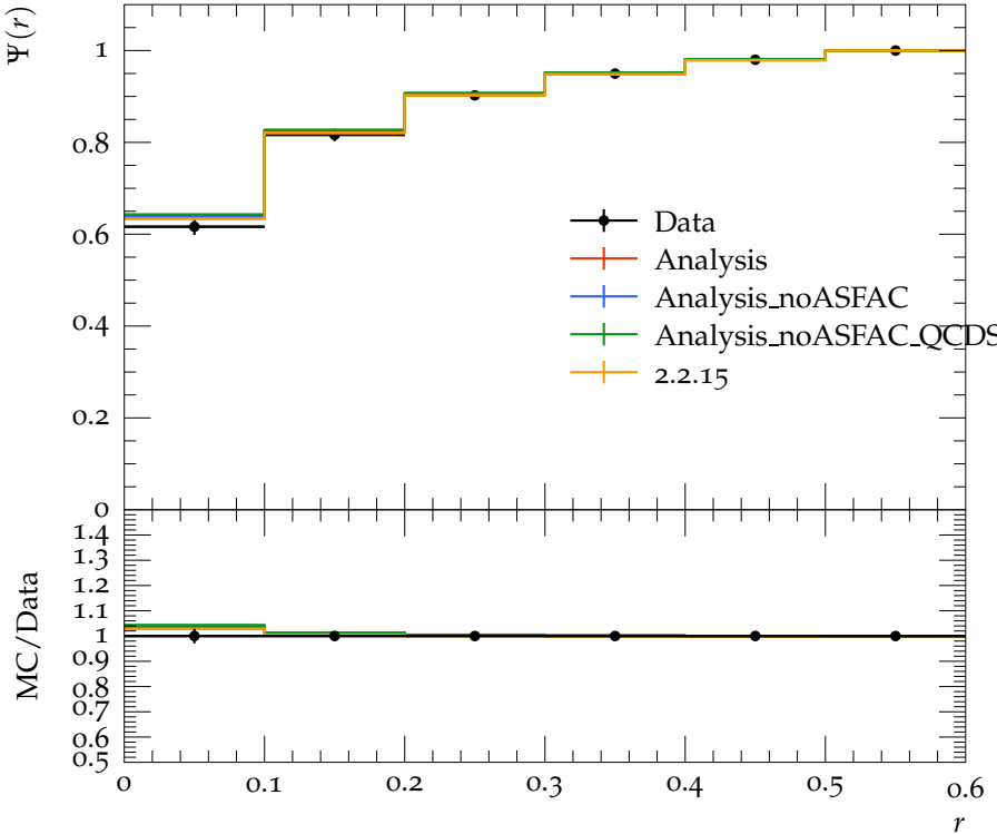
Jet shape \Psi for p_{\perp} \in 110\text{--}160\text{ GeV} , y \in 0.8\text{--}1.2
