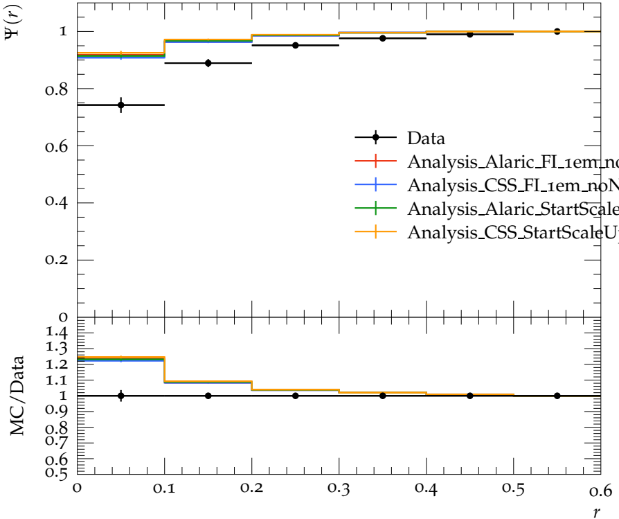
Jet shape \Psi for p_{\perp} \in 400\text{--}500\text{ GeV} , y \in 0.0\text{--}0.3
