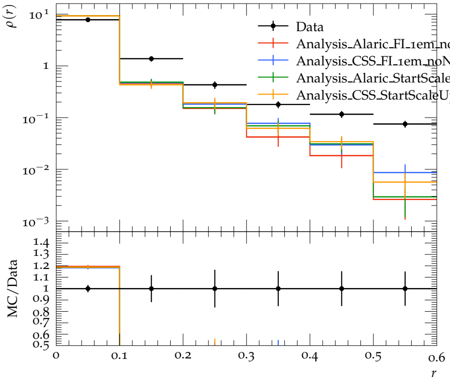
Jet shape \rho for p_{\perp} \in 400\text{--}500\text{ GeV} , y \in 0.3\text{--}0.8
