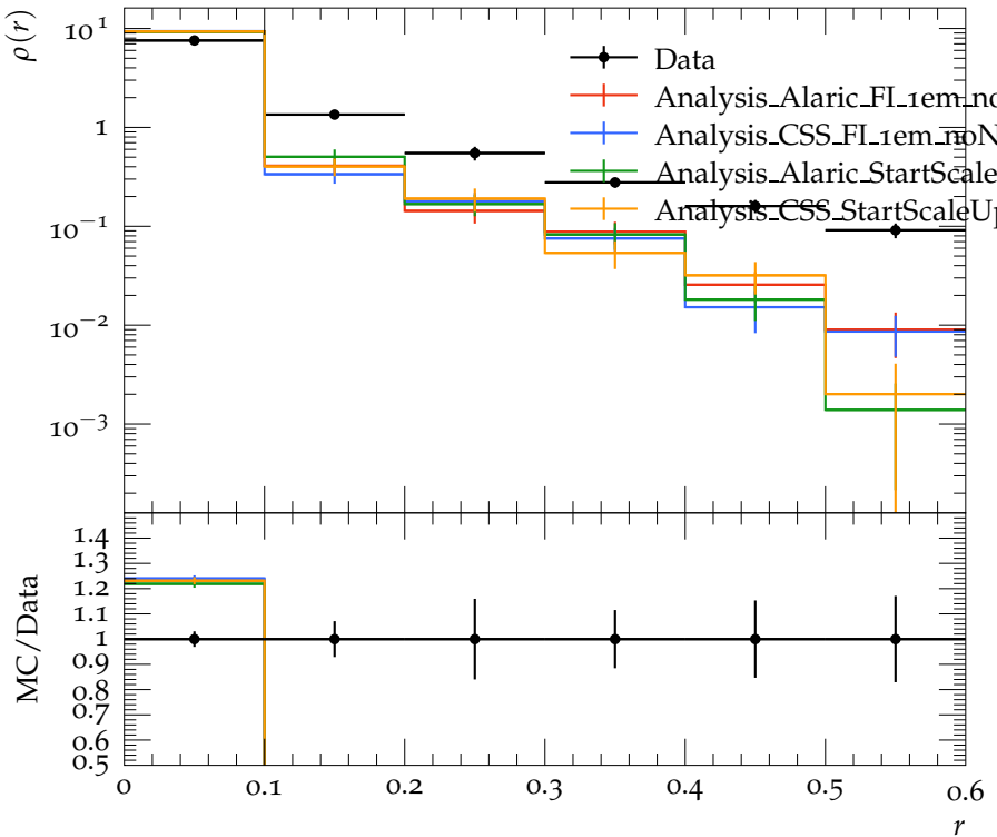
Jet shape \rho for p_{\perp} \in 310\text{--}400 GeV, y \in 0.8\text{--}1.2
