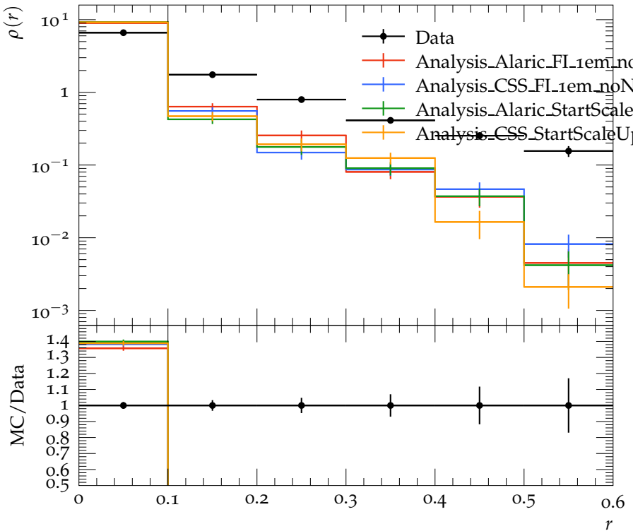
Jet shape \rho for p_{\perp} \in 160\text{--}210\text{ GeV} , y \in 0.8\text{--}1.2
