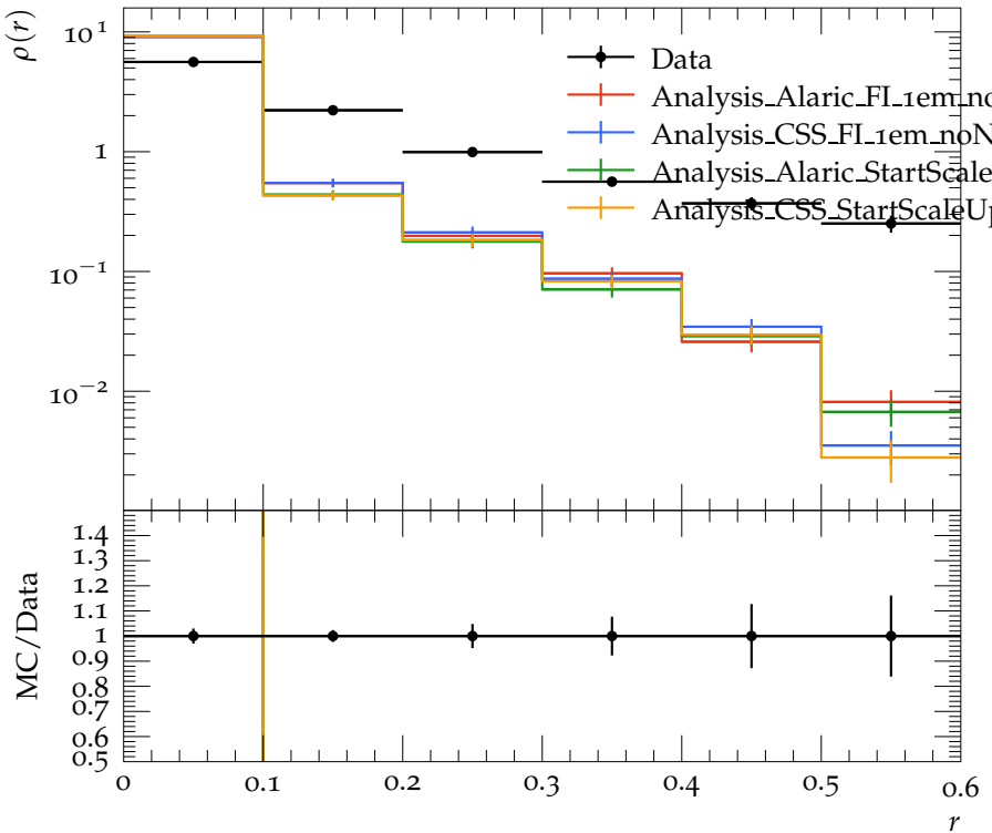
Jet shape \rho for p_{\perp} \in 80\text{--}110\text{ GeV} , y \in 0.3\text{--}0.8
