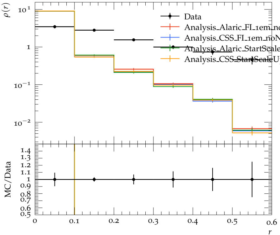
Jet shape \rho for p_{\perp} \in 30\text{--}40\text{ GeV} , y \in 0.8\text{--}1.2
