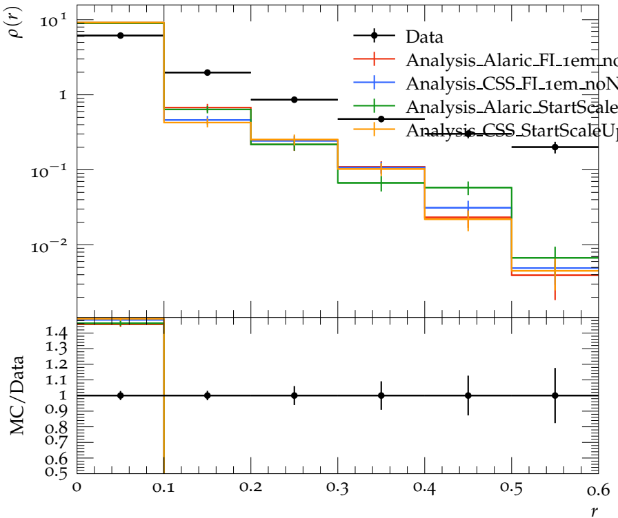
Jet shape \rho for p_{\perp} \in 110\text{--}160\text{ GeV} , y \in 0.8\text{--}1.2
