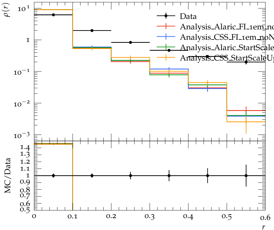
Jet shape \rho for p_{\perp} \in 110\text{--}160\text{ GeV} , y \in 0.3\text{--}0.8
