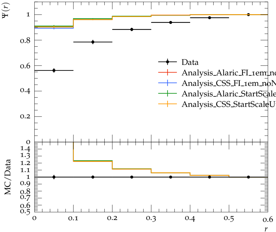
Jet shape \Psi for p_{\perp} \in 80\text{--}110\text{ GeV} , y \in 0.8\text{--}1.2
