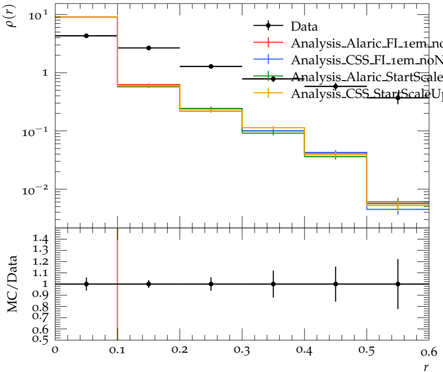
Jet shape \rho for p_{\perp} \in 40\text{--}60\text{ GeV} , y \in 0.8\text{--}1.2
