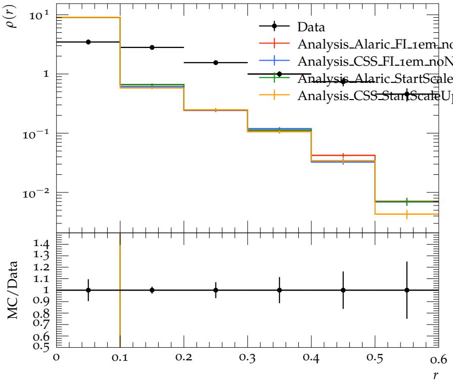
Jet shape \rho for p_{\perp} \in 30\text{--}40\text{ GeV} , y \in 0.8\text{--}1.2
