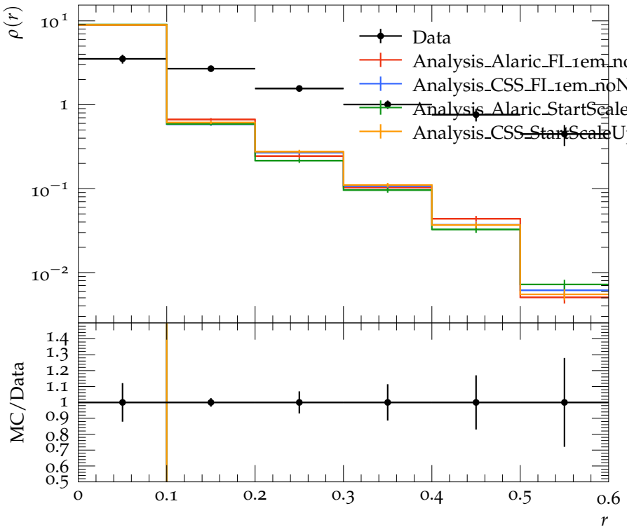
Jet shape \rho for p_{\perp} \in 30\text{--}40\text{ GeV} , y \in 0.3\text{--}0.8
