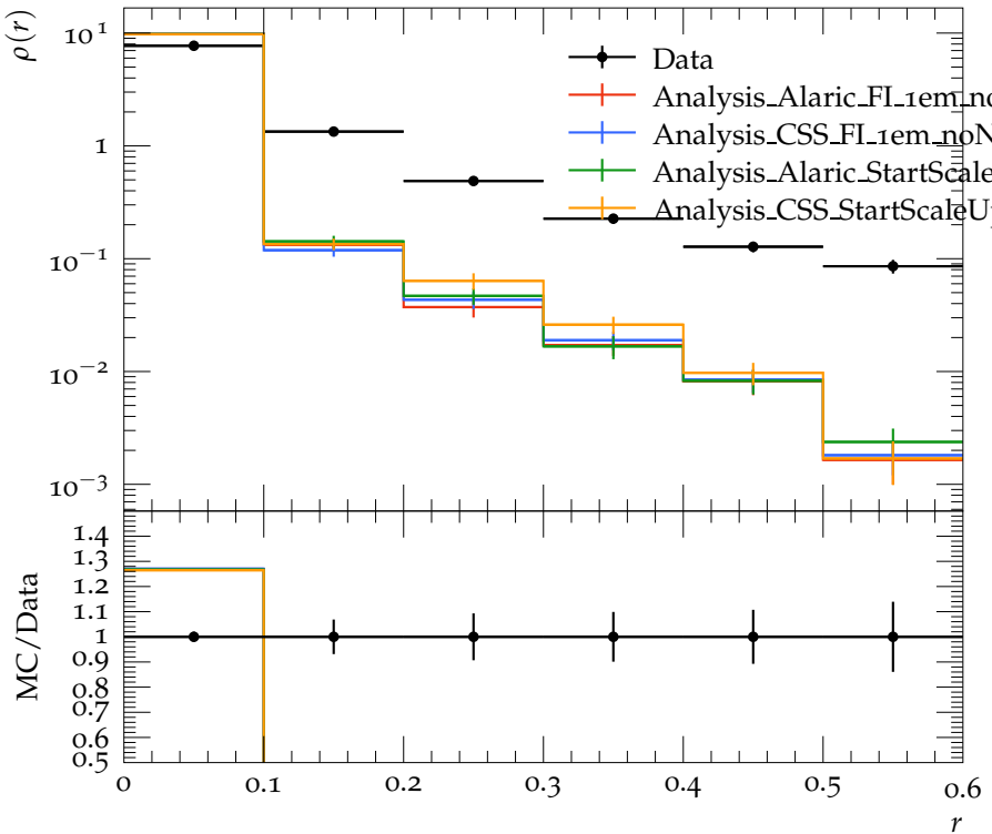
Jet shape \rho for p_{\perp} \in 400\text{--}500\text{ GeV} , y \in 0.0\text{--}2.8
