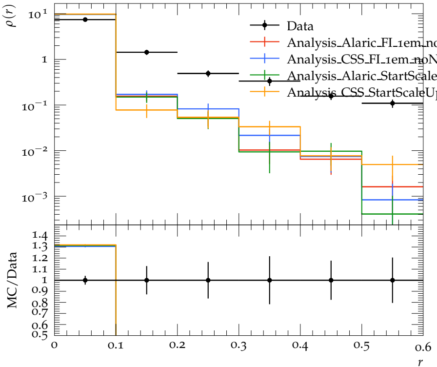
Jet shape \rho for p_{\perp} \in 400\text{--}500\text{ GeV} , y \in 0.8\text{--}1.2
