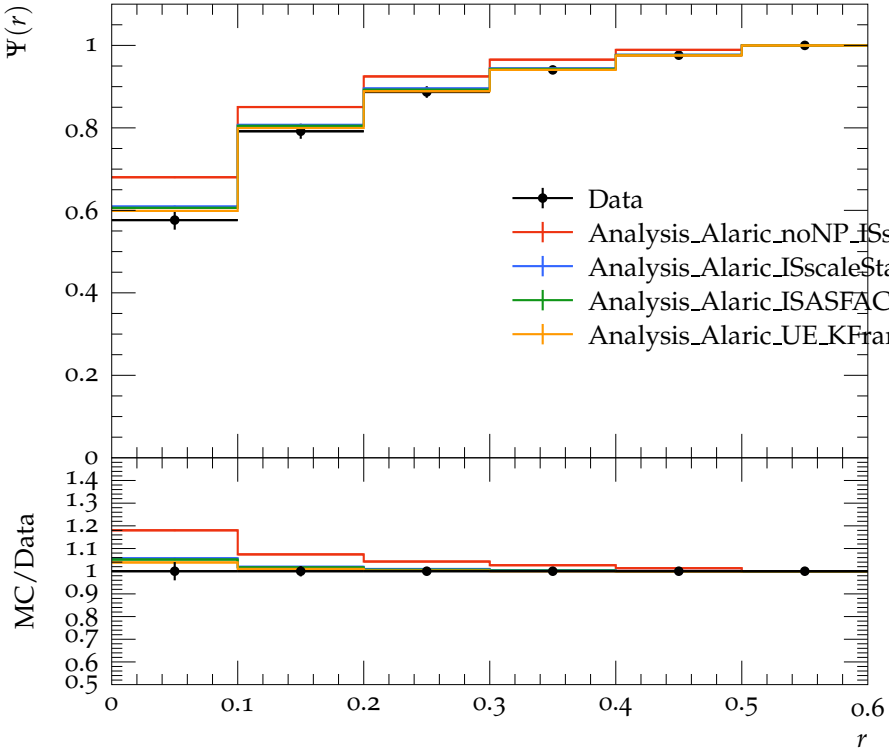
Jet shape \Psi for p_{\perp} \in 80\text{--}110\text{ GeV} , y \in 1.2\text{--}2.1
