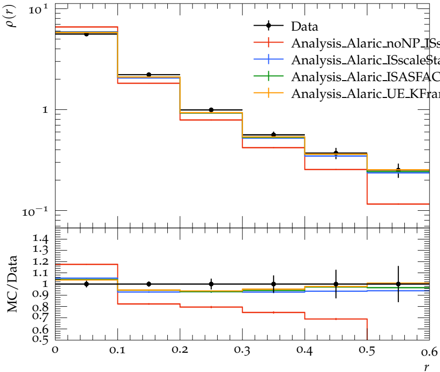
Jet shape \rho for p_{\perp} \in 80\text{--}110\text{ GeV} , y \in 0.3\text{--}0.8
