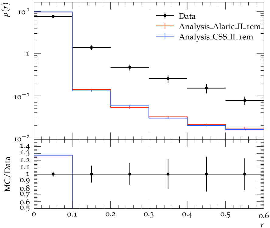
Jet shape \rho for p_{\perp} \in 500\text{--}600\text{ GeV} , y \in 0.0\text{--}2.8
