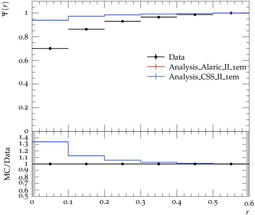
Jet shape \Psi for p_{\perp} \in 210\text{--}260\text{ GeV} , y \in 0.0\text{--}2.8
