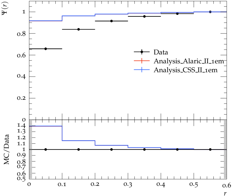
Jet shape \Psi for p_{\perp} \in 160\text{--}210\text{ GeV} , y \in 0.3\text{--}0.8
