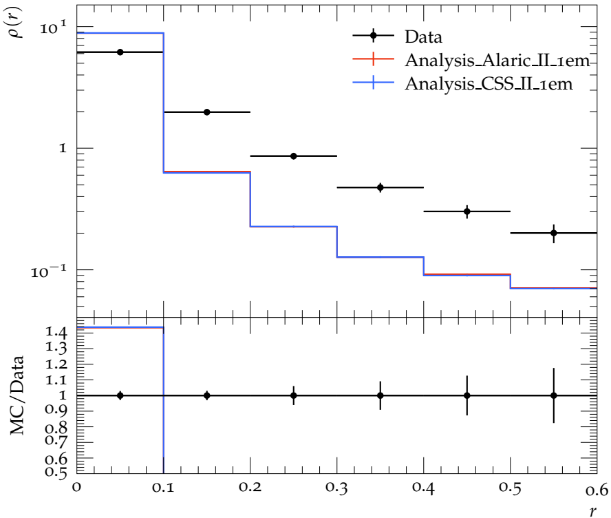
Jet shape \rho for p_{\perp} \in 110\text{--}160\text{ GeV} , y \in 0.8\text{--}1.2
