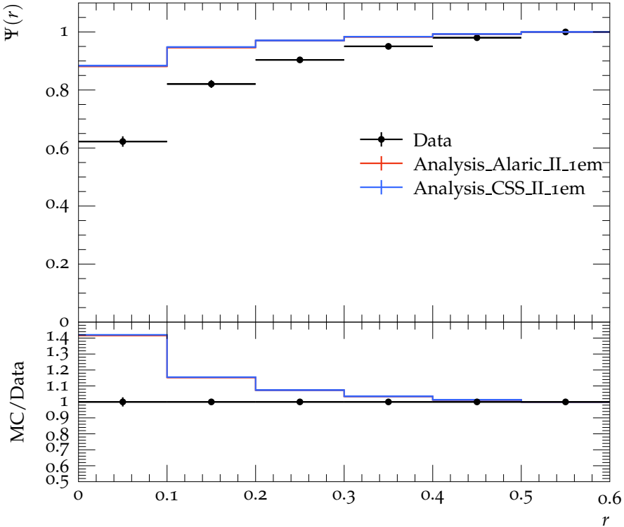
Jet shape \Psi for p_{\perp} \in 110\text{--}160\text{ GeV} , y \in 0.3\text{--}0.8
