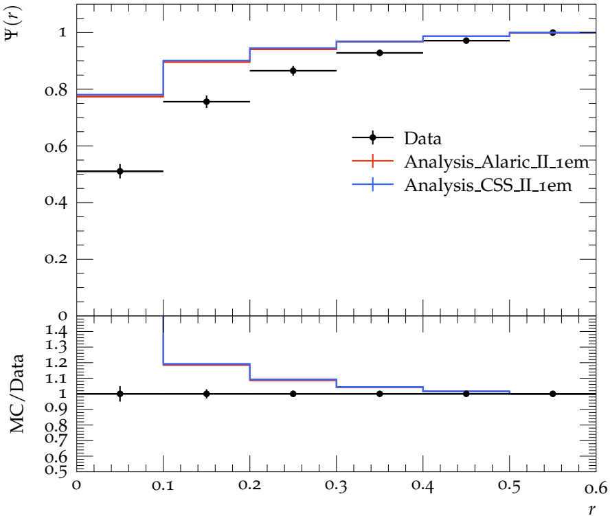
Jet shape \Psi for p_{\perp} \in 60\text{--}80\text{ GeV} , y \in 0.8\text{--}1.2
