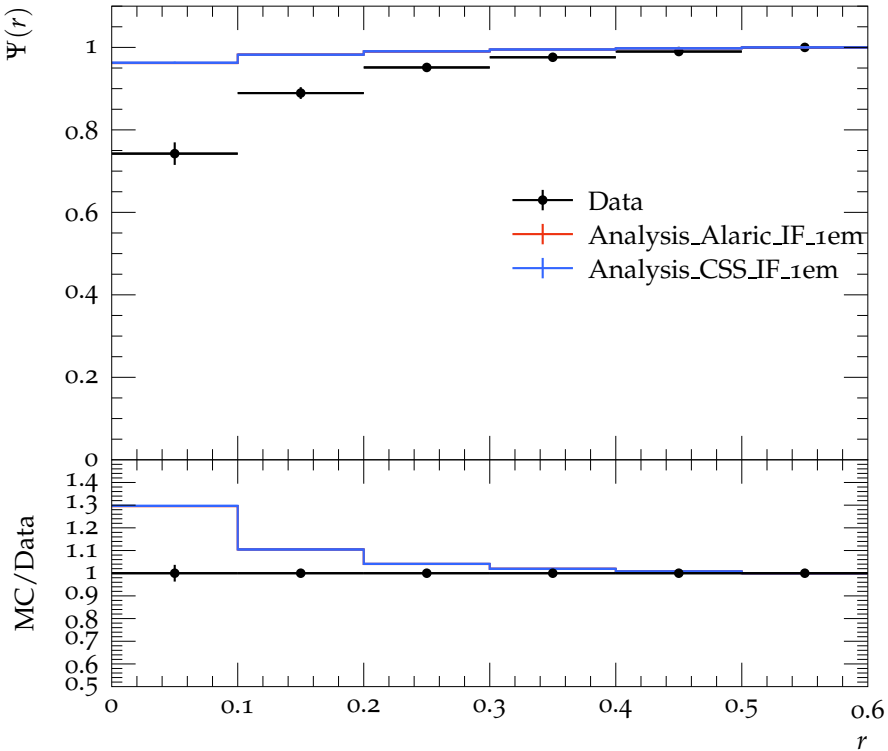
Jet shape \Psi for p_{\perp} \in 400\text{--}500\text{ GeV} , y \in 0.0\text{--}0.3
