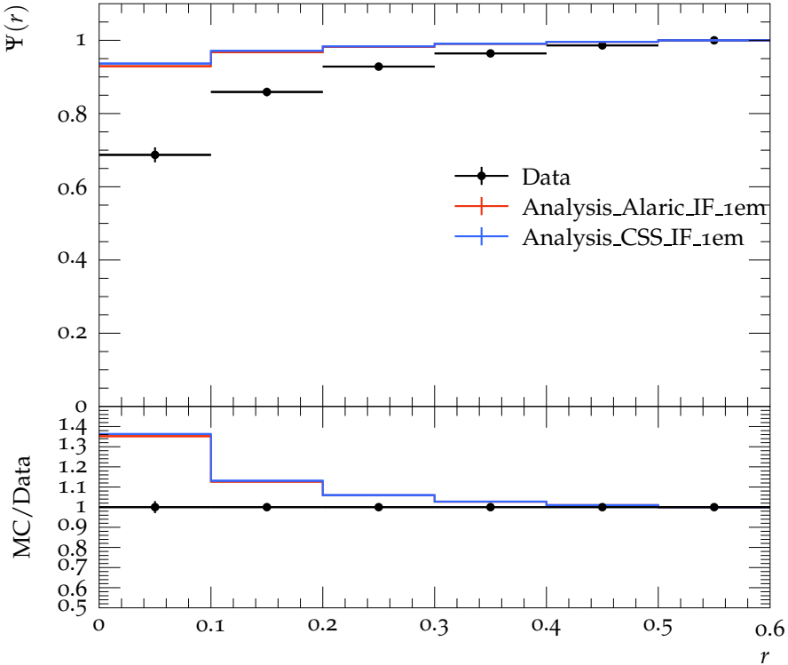
Jet shape \Psi for p_{\perp} \in 210\text{--}260\text{ GeV} , y \in 0.3\text{--}0.8
