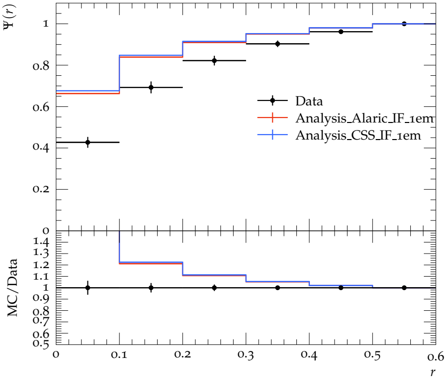
Jet shape \Psi for p_{\perp} \in 40\text{--}60\text{ GeV} , y \in 0.3\text{--}0.8
