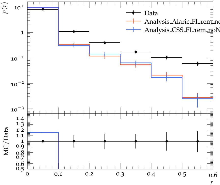
Jet shape \rho for p_{\perp} \in 400\text{--}500\text{ GeV} , y \in 1.2\text{--}2.1
