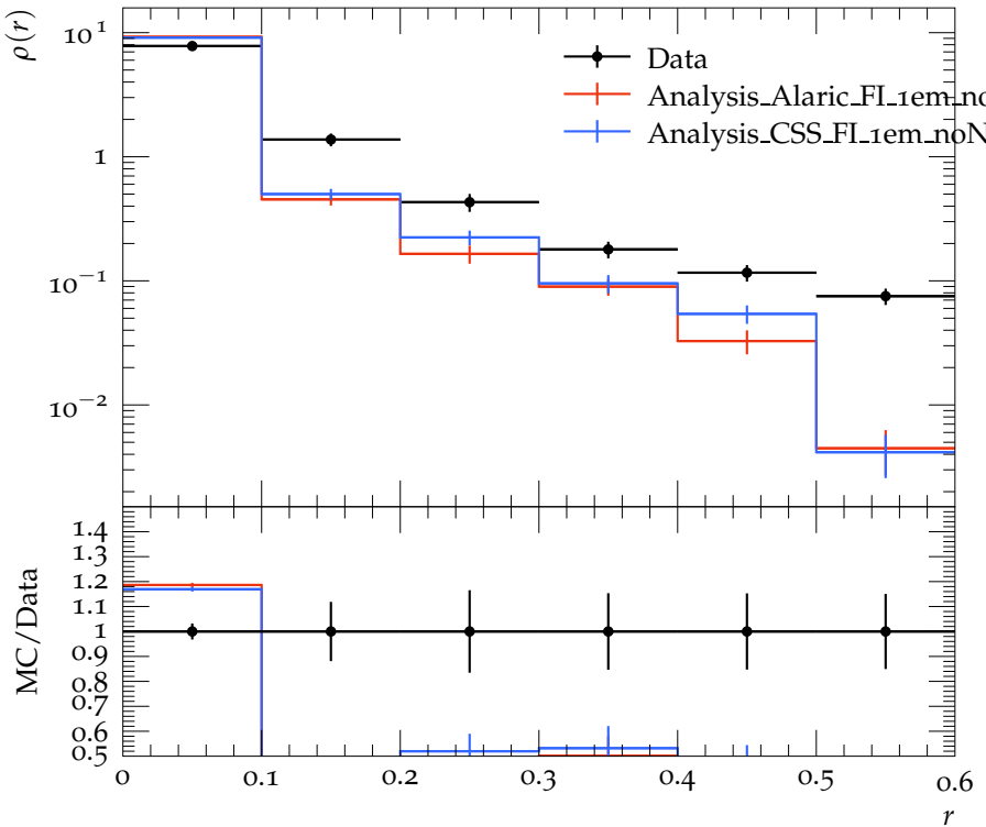
Jet shape \rho for p_{\perp} \in 400\text{--}500\text{ GeV} , y \in 0.3\text{--}0.8
