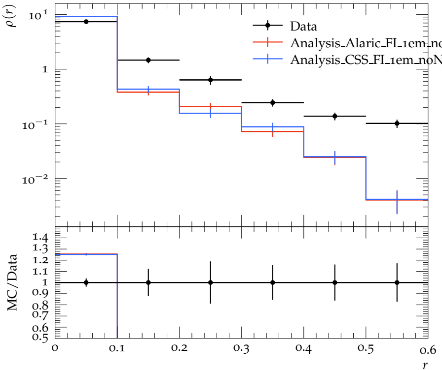
Jet shape \rho for p_{\perp} \in 400\text{--}500\text{ GeV} , y \in 0.0\text{--}0.3
