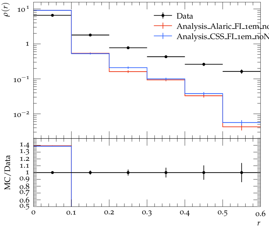
Jet shape \rho for p_{\perp} \in 160\text{--}210\text{ GeV} , y \in 0.3\text{--}0.8
