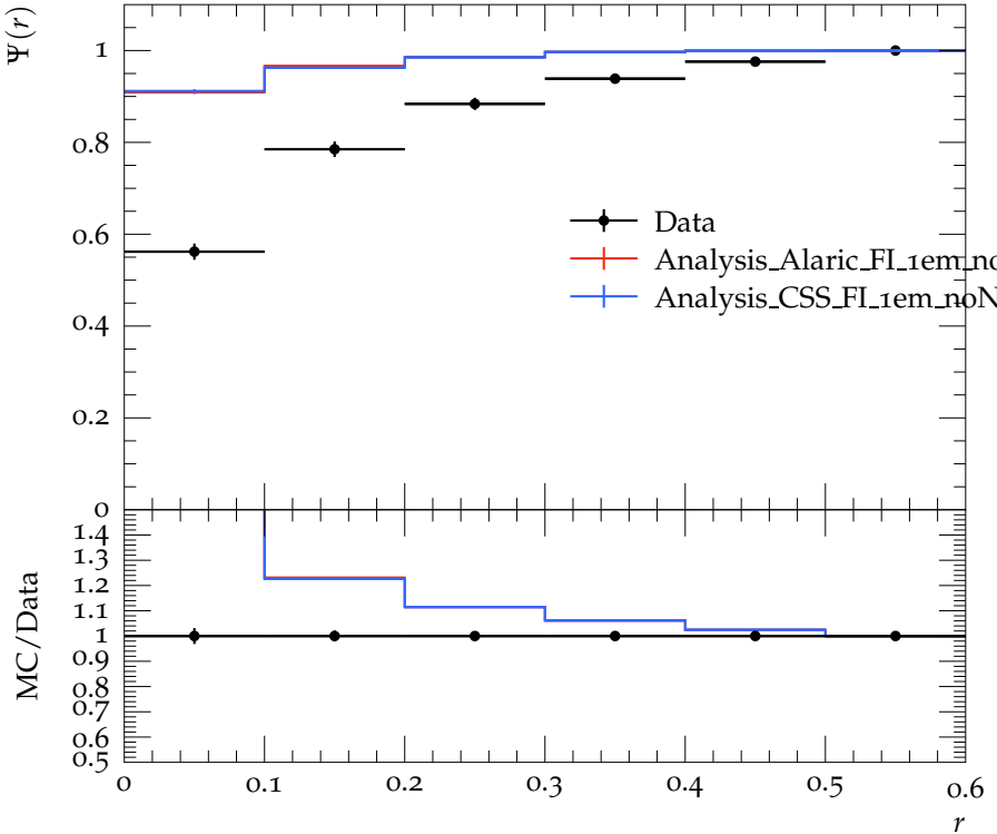
Jet shape \Psi for p_{\perp} \in 80\text{--}110\text{ GeV} , y \in 0.8\text{--}1.2
