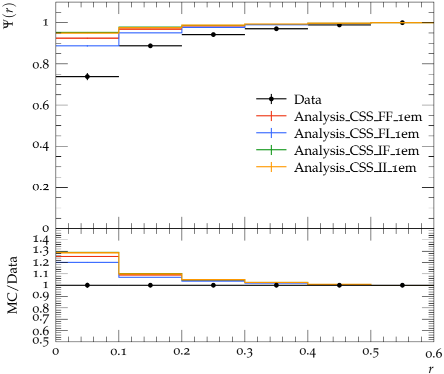
Jet shape \Psi for p_{\perp} \in 310\text{--}400\text{ GeV} , y \in 0.0\text{--}0.3
