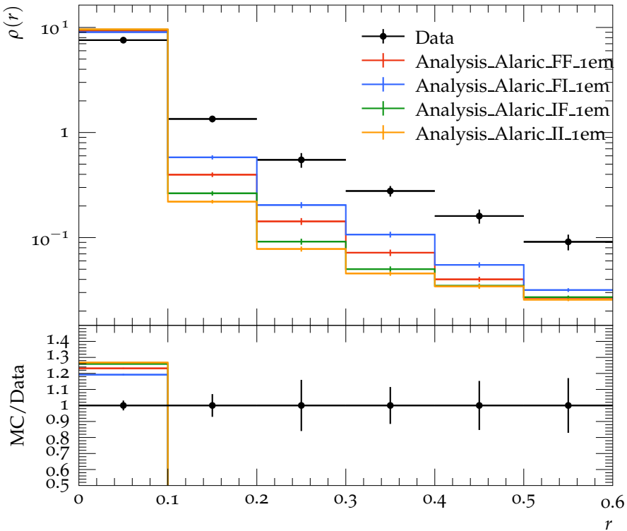
Jet shape \rho for p_{\perp} \in 310\text{--}400 GeV, y \in 0.8\text{--}1.2
