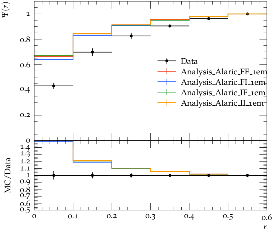
Jet shape \Psi for p_{\perp} \in 40\text{--}60\text{ GeV} , y \in 0.8\text{--}1.2
