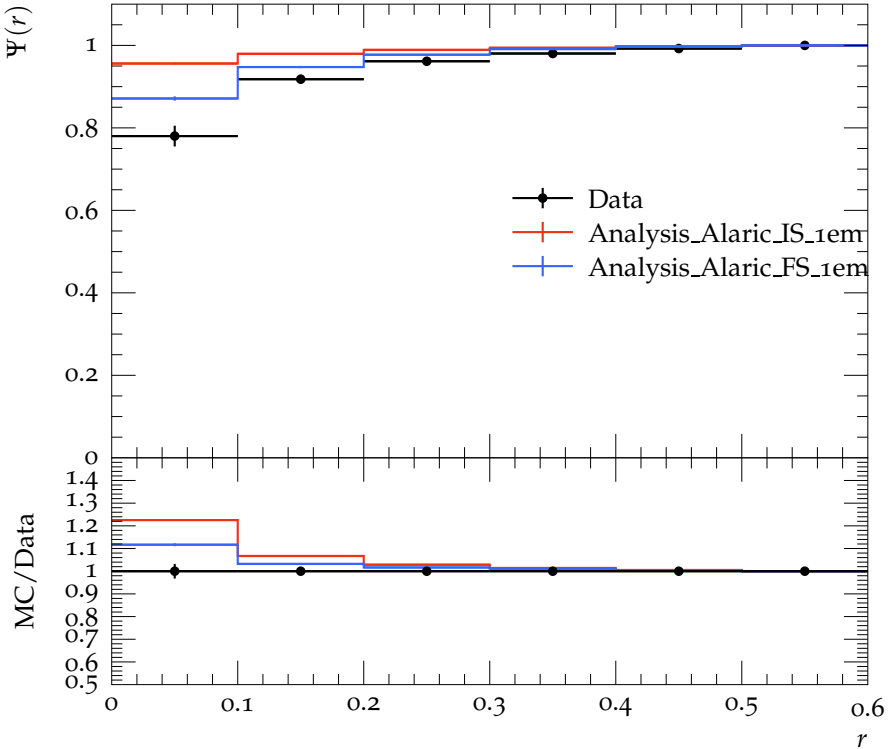
Jet shape \Psi for p_{\perp} \in 400\text{--}500\text{ GeV} , y \in 0.3\text{--}0.8
