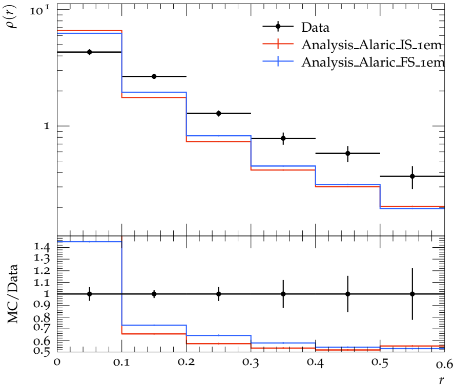
Jet shape \rho for p_{\perp} \in 40\text{--}60\text{ GeV} , y \in 0.8\text{--}1.2
