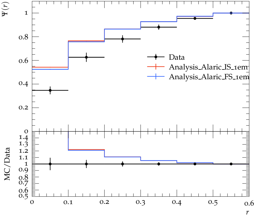
Jet shape \Psi for p_{\perp} \in 30\text{--}40\text{ GeV} , y \in 0.8\text{--}1.2
