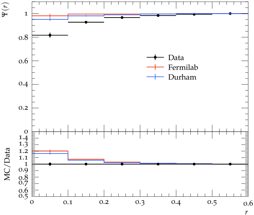
Jet shape \Psi for p_{\perp} \in 400\text{--}500\text{ GeV} , y \in 1.2\text{--}2.1
