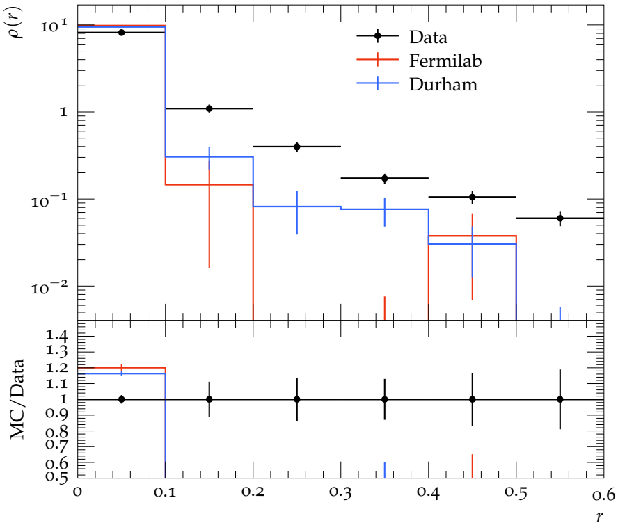
Jet shape \rho for p_{\perp} \in 400\text{--}500\text{ GeV} , y \in 1.2\text{--}2.1
