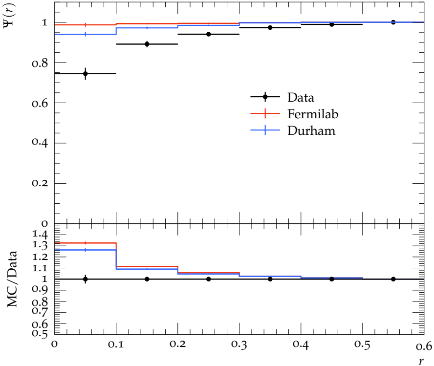
Jet shape \Psi for p_{\perp} \in 400\text{--}500\text{ GeV} , y \in 0.8\text{--}1.2
