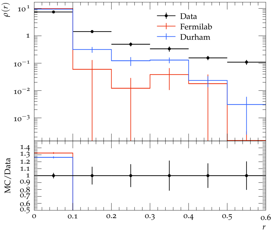
Jet shape \rho for p_{\perp} \in 400\text{--}500\text{ GeV} , y \in 0.8\text{--}1.2
