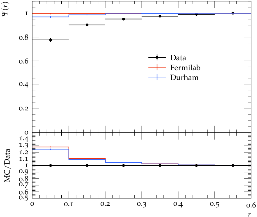
Jet shape \Psi for p_{\perp} \in 310\text{--}400\text{ GeV} , y \in 1.2\text{--}2.1
