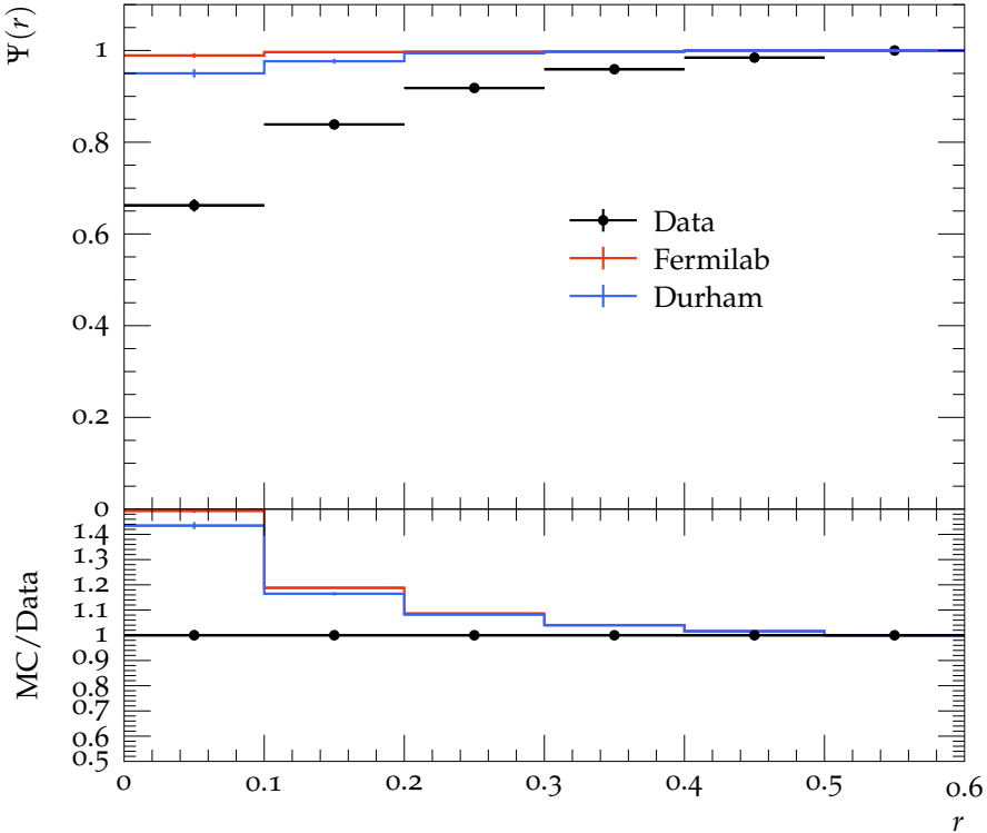
Jet shape \Psi for p_{\perp} \in 160\text{--}210\text{ GeV} , y \in 0.8\text{--}1.2
