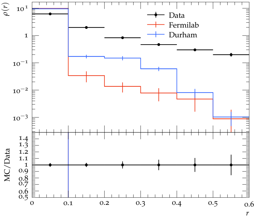
Jet shape \rho for p_{\perp} \in 110\text{--}160\text{ GeV} , y \in 0.3\text{--}0.8
