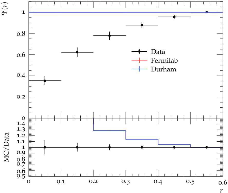
Jet shape \Psi for p_{\perp} \in 30\text{--}40\text{ GeV} , y \in 0.3\text{--}0.8
