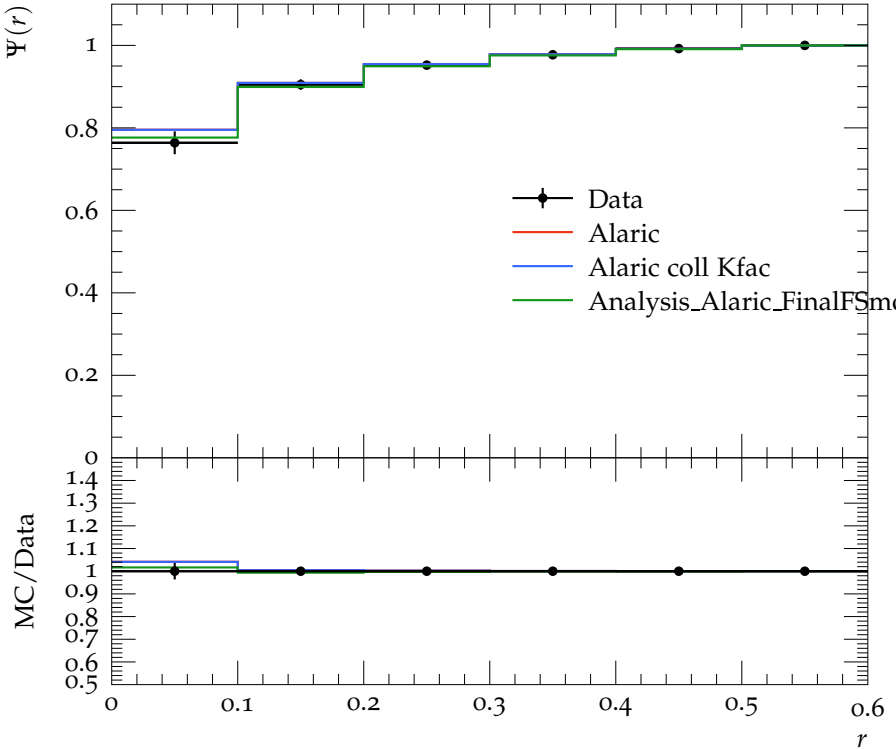
Jet shape \Psi for p_{\perp} \in 500\text{--}600\text{ GeV} , y \in 0.0\text{--}2.8
