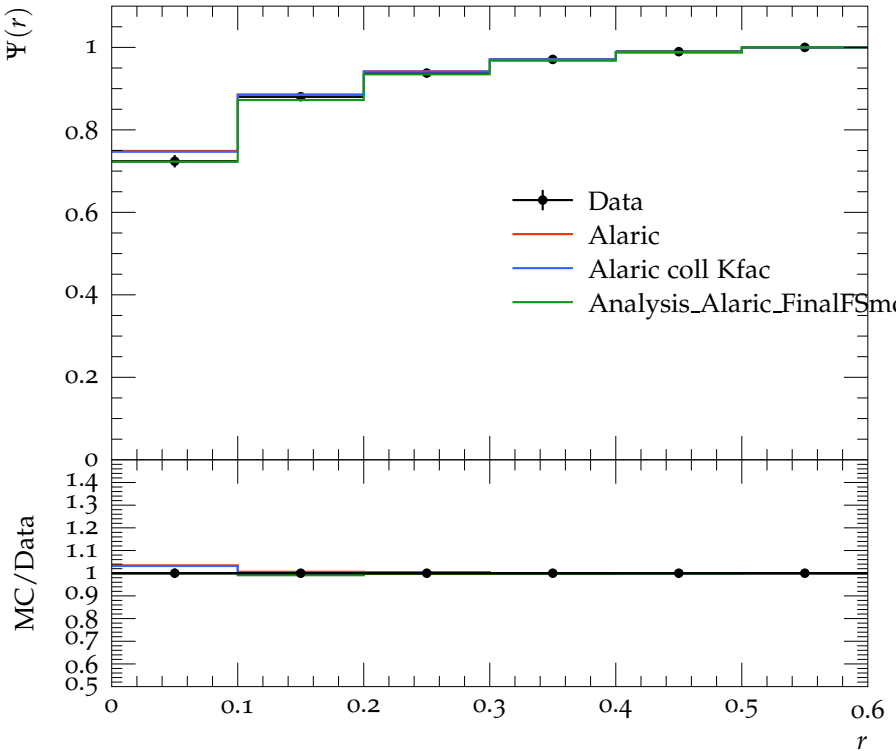
Jet shape \Psi for p_{\perp} \in 310\text{--}400\text{ GeV} , y \in 0.3\text{--}0.8
