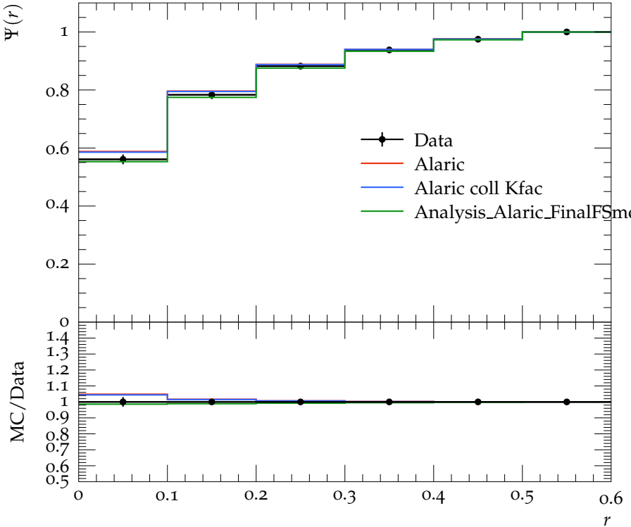
Jet shape \Psi for p_{\perp} \in 80\text{--}110\text{ GeV} , y \in 0.3\text{--}0.8
